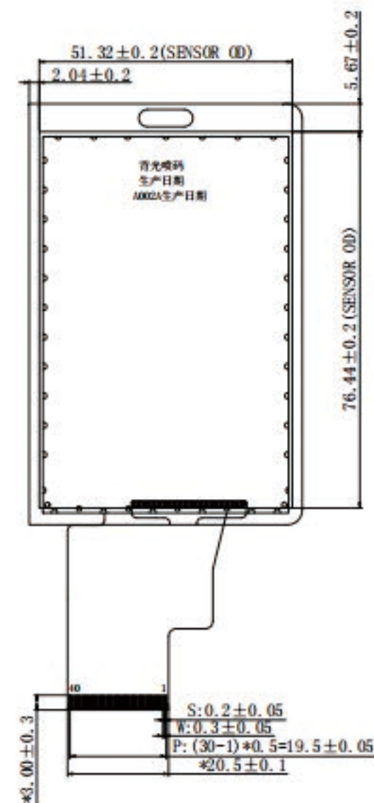
背视图
